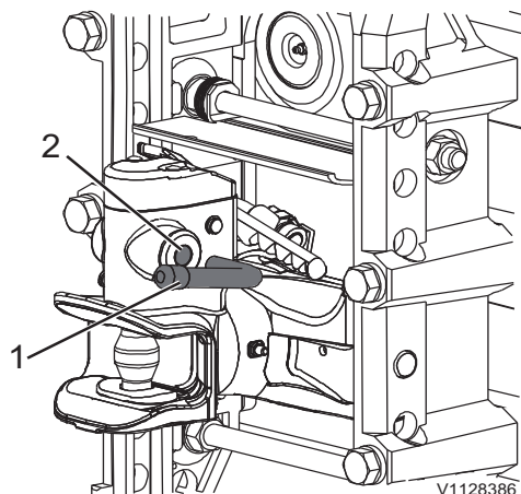
Trekhaak stempelhouder
